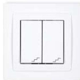
Łącznik podwójny schodowy + ramka uniwersalna pojedyncza z tworzywa / Double two-way switch + 1-gang universal plastic frame DWP-33 + DR-1
